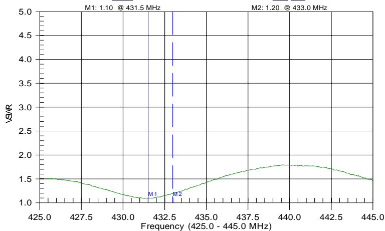
VSWR MIN 433MHZ
